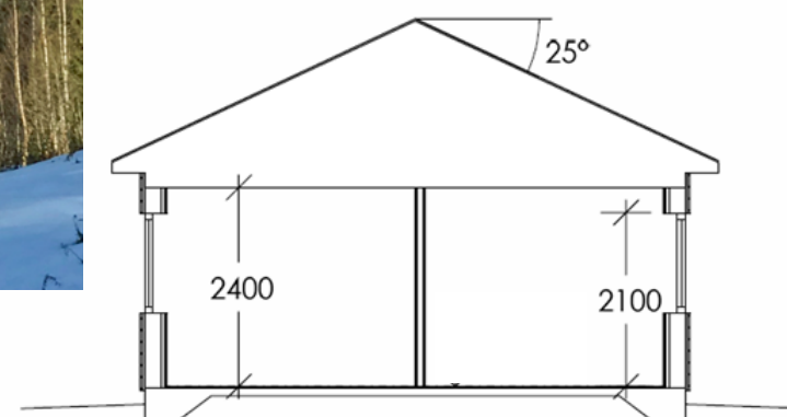
SEKTION A-A 1:100/A3
