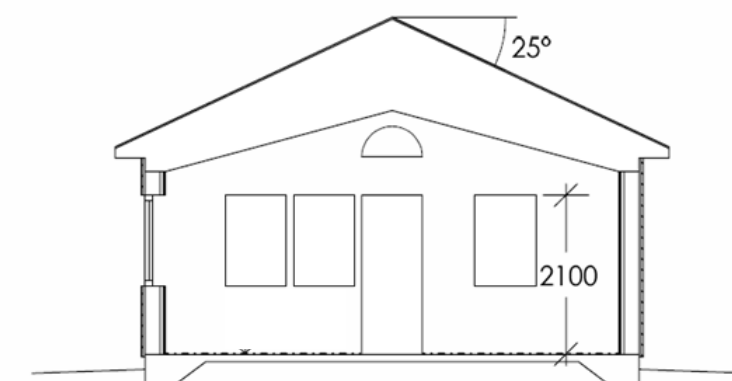
SEKTION B-B 1:100/A3
